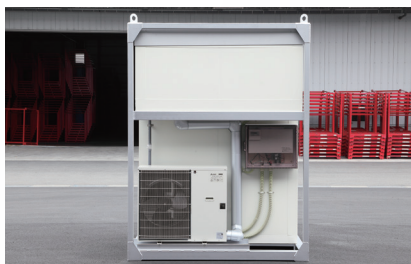
冷凍機(外観)
