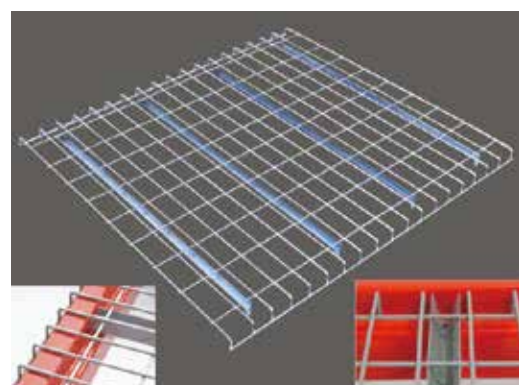
S型 (Step Style) パレット
